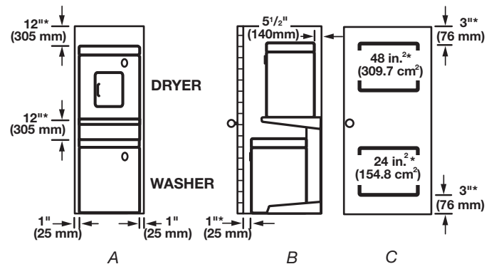
A. Encastrement B. Vue latérale – placard ou endroit exigu C. Porte du placard avec grilles d'aération
