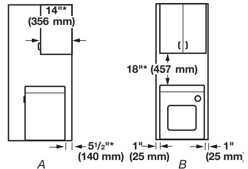
A. Vue latérale – placard ou endroit exigu B. Zone d'insertion
