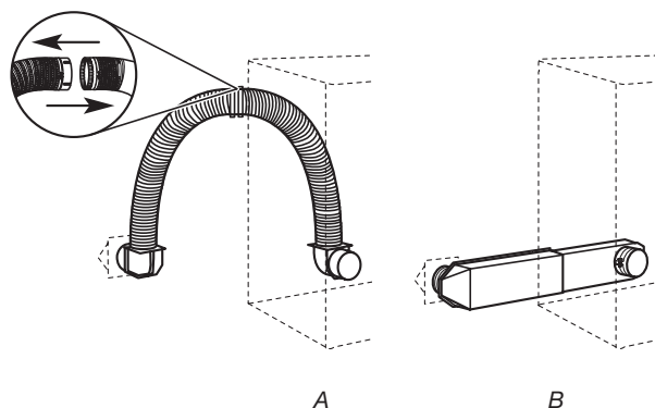
A. Installation au-dessus de la sécheuse (également disponible avec un coude décalé) B. Installation de périscope
