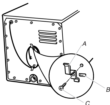
A. Support du cordon B. Fente C. Vis
